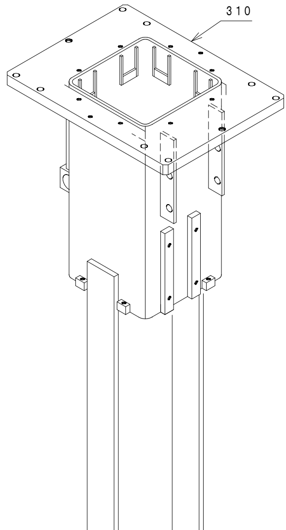
「A」矢視図
