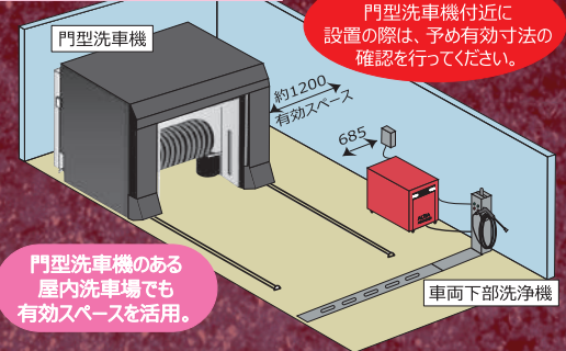
自動下部洗浄装置 JR-54 CS9002-0001
