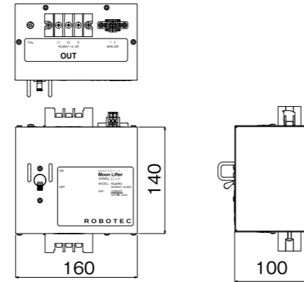
非常停止ユニット (200V)
