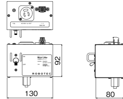
非常停止ユニット (100V)
