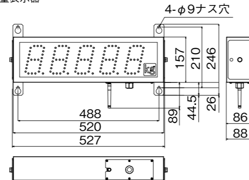
大型重量表示器
